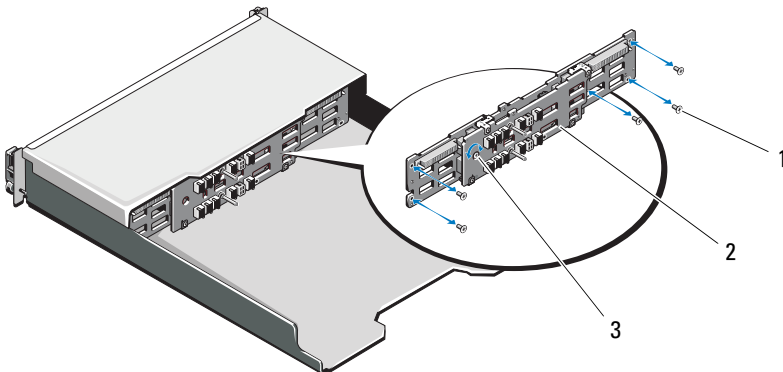
Abbildung 3-14. Entfernen und Installieren der Rückwandplatine – PowerVault MD1200
