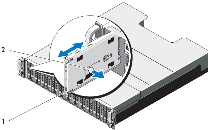
Abbildung 3-12. Entfernen und Installieren der Bedienfeldplatte – PowerVault MD1220
