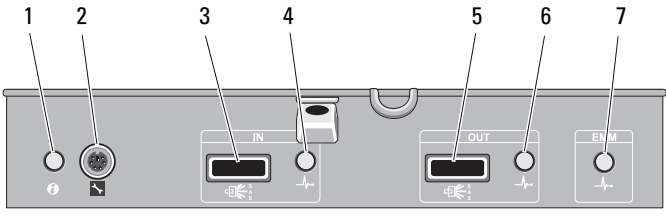
Abbildung 1-6. Gehäuseverwaltungsmodul (EMM)
